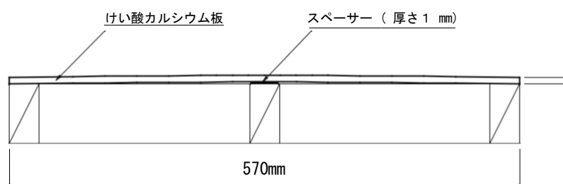
図 5 下地の断面図 (図 4 の A-A 断面)
