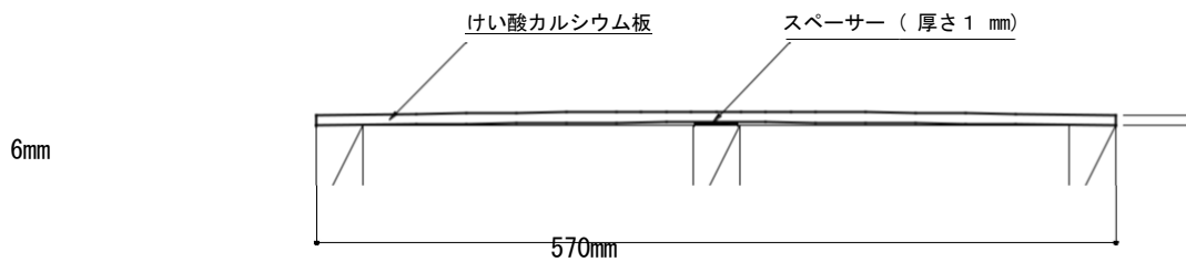
図 1 下地の断面図 (図 1 の A-A 断面)
