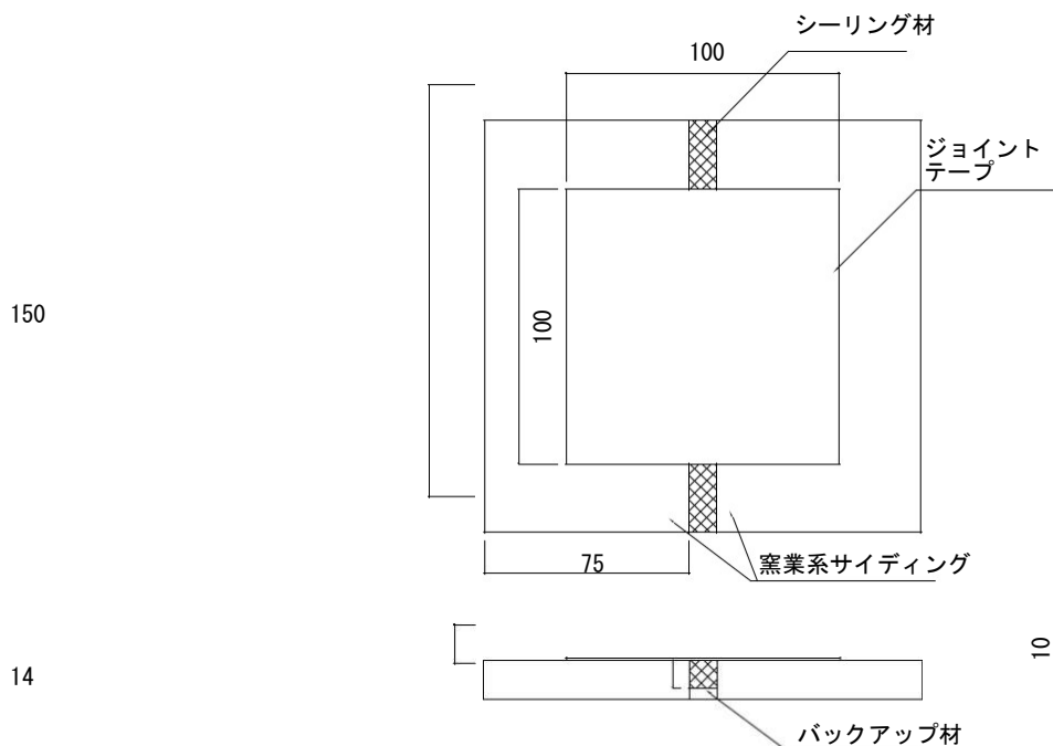
図 1 試料の作製および検査方法
