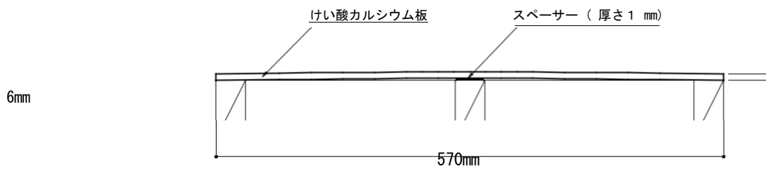
図 2 下地の断面図 (図 1 の A-A 断面)
