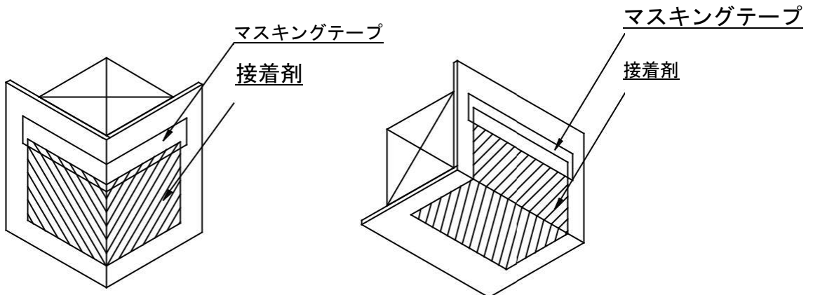
図 3 接着剤の塗布（出隅の場合）
