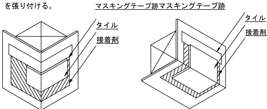
図 5 タイルの張り付け（出隅の場合）
