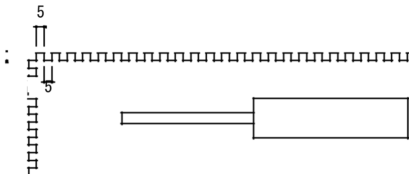
図 1 標準くし目こて
